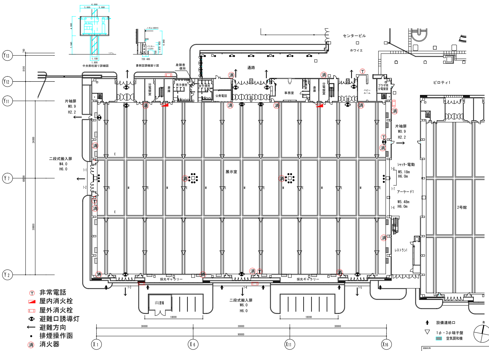
図面名称 1号館 1階平面図
