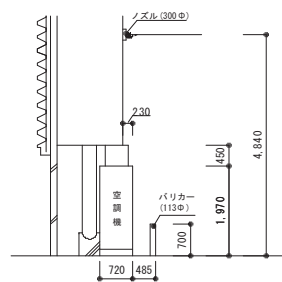
壁側空調機廻り図
